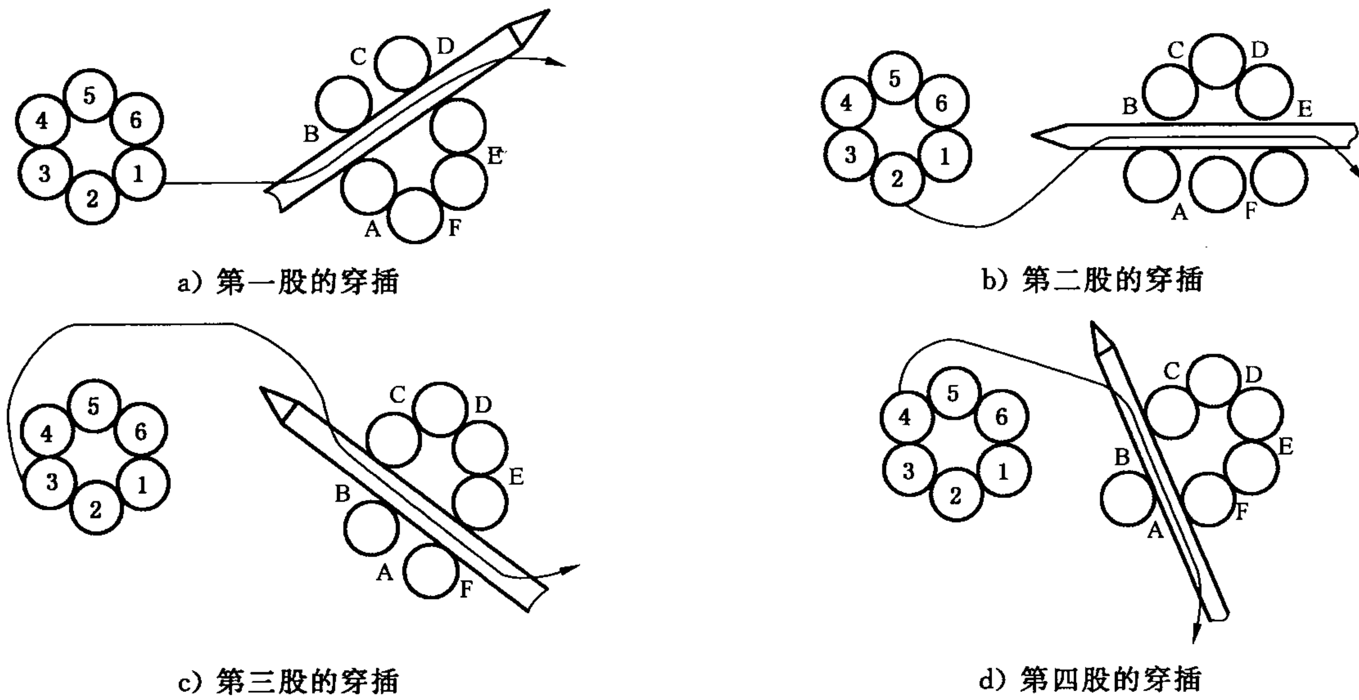
图 A.2 手工插编初期的方法
