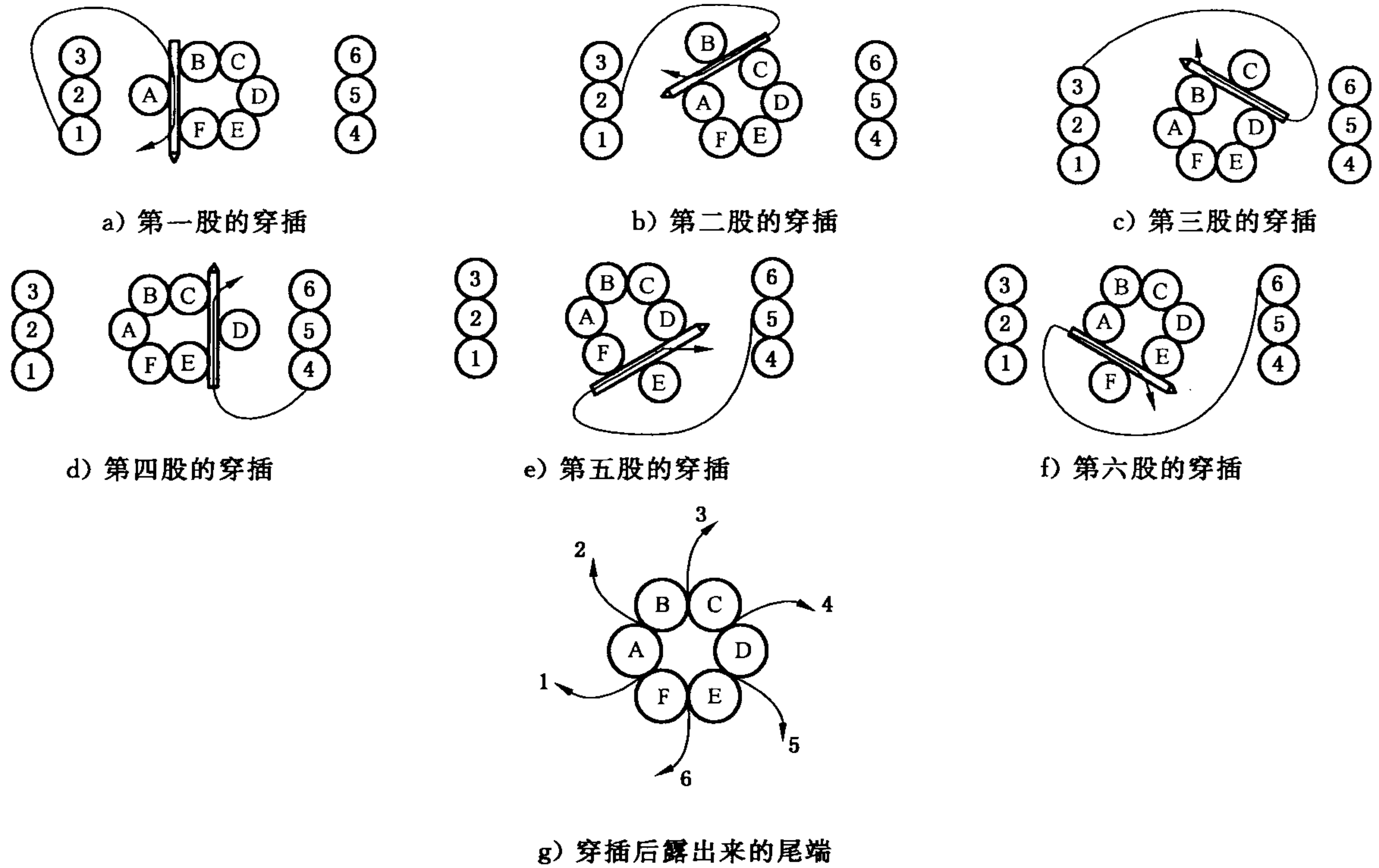
图 B.4 手工插编方法
