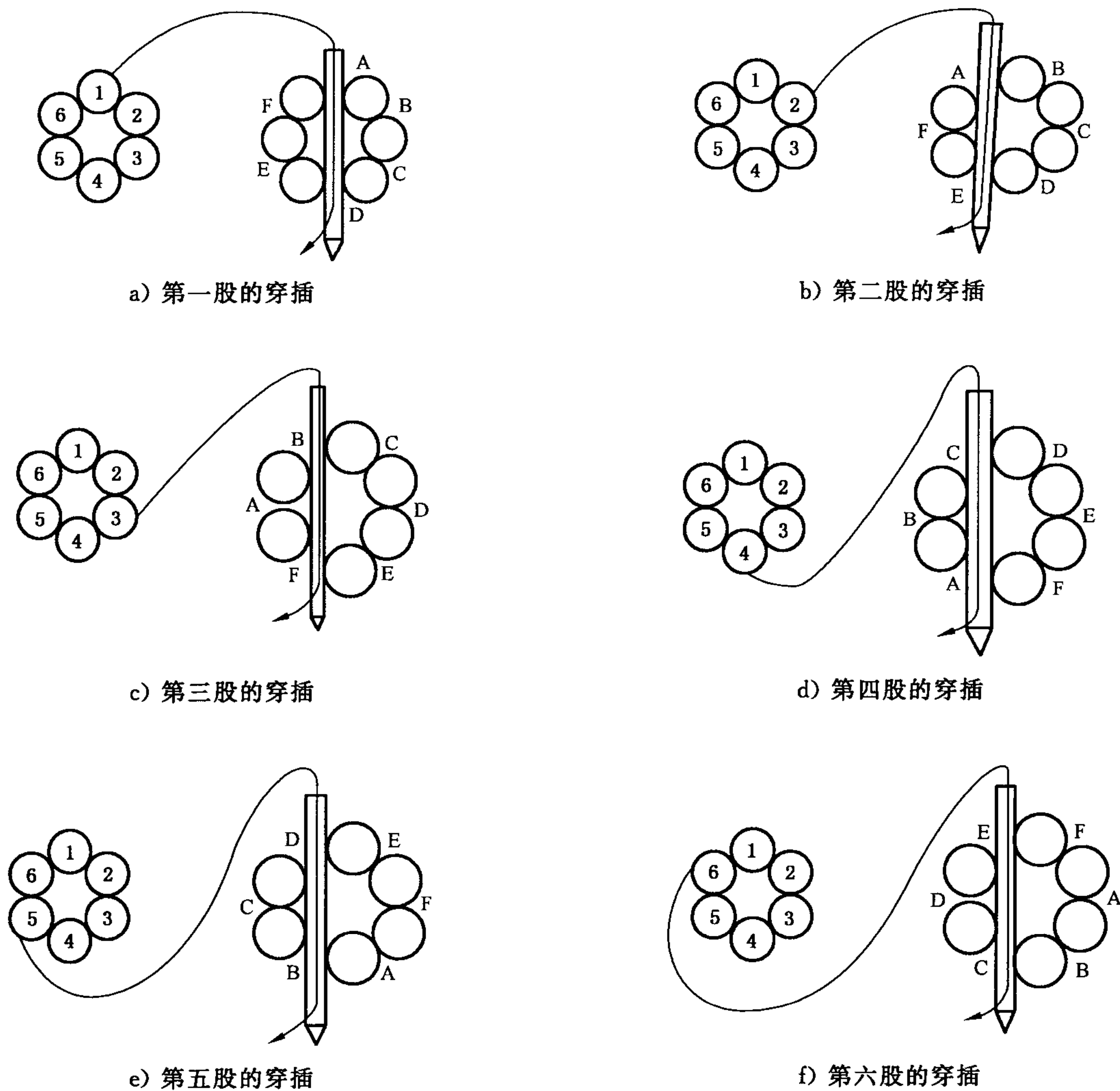
图 C.1 机械插编初期的方法
