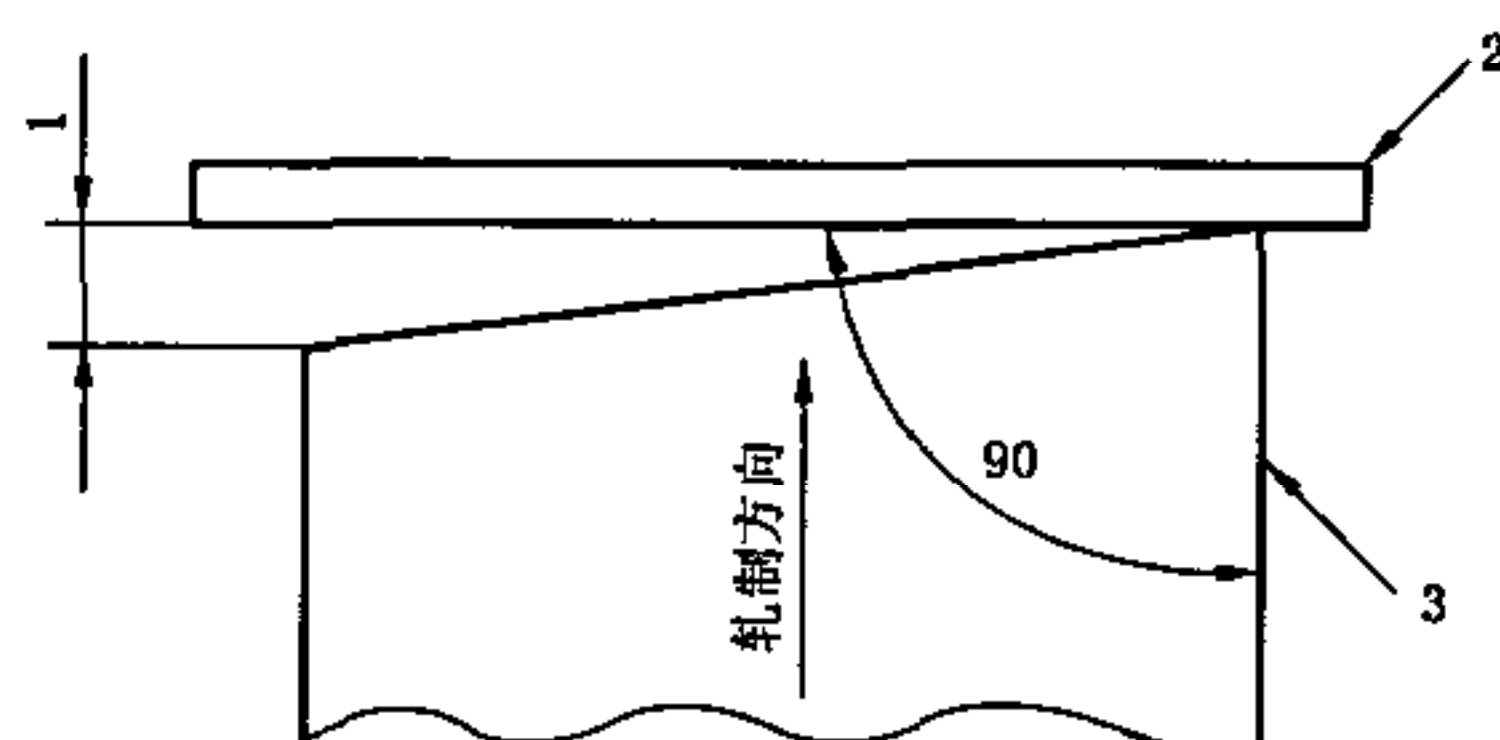
图 3 镰刀弯的测量
