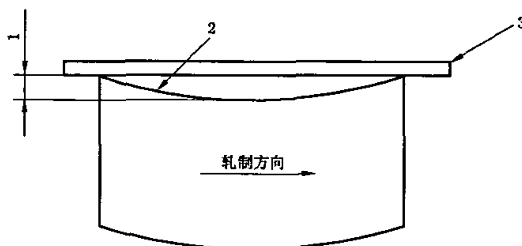
图 2 连轧钢板不平度的测量
