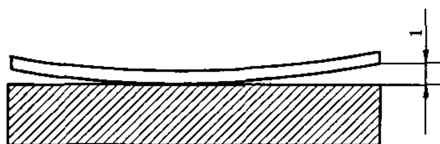
图 2 连轧钢板不平度的测量
