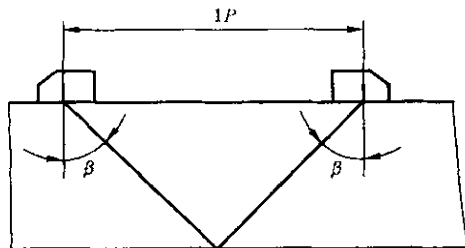
图 C1 灵敏度调节
