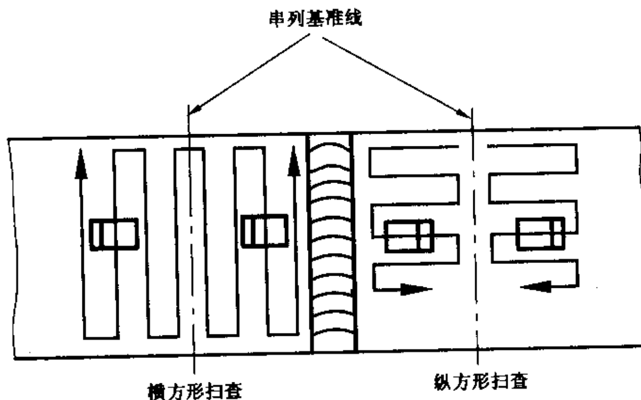
图 4 横方形扫查及纵方形扫查
