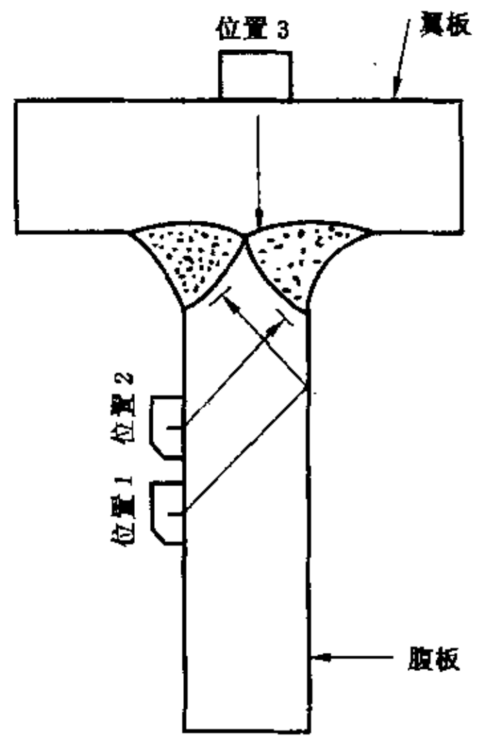
图 16 T 型接头
