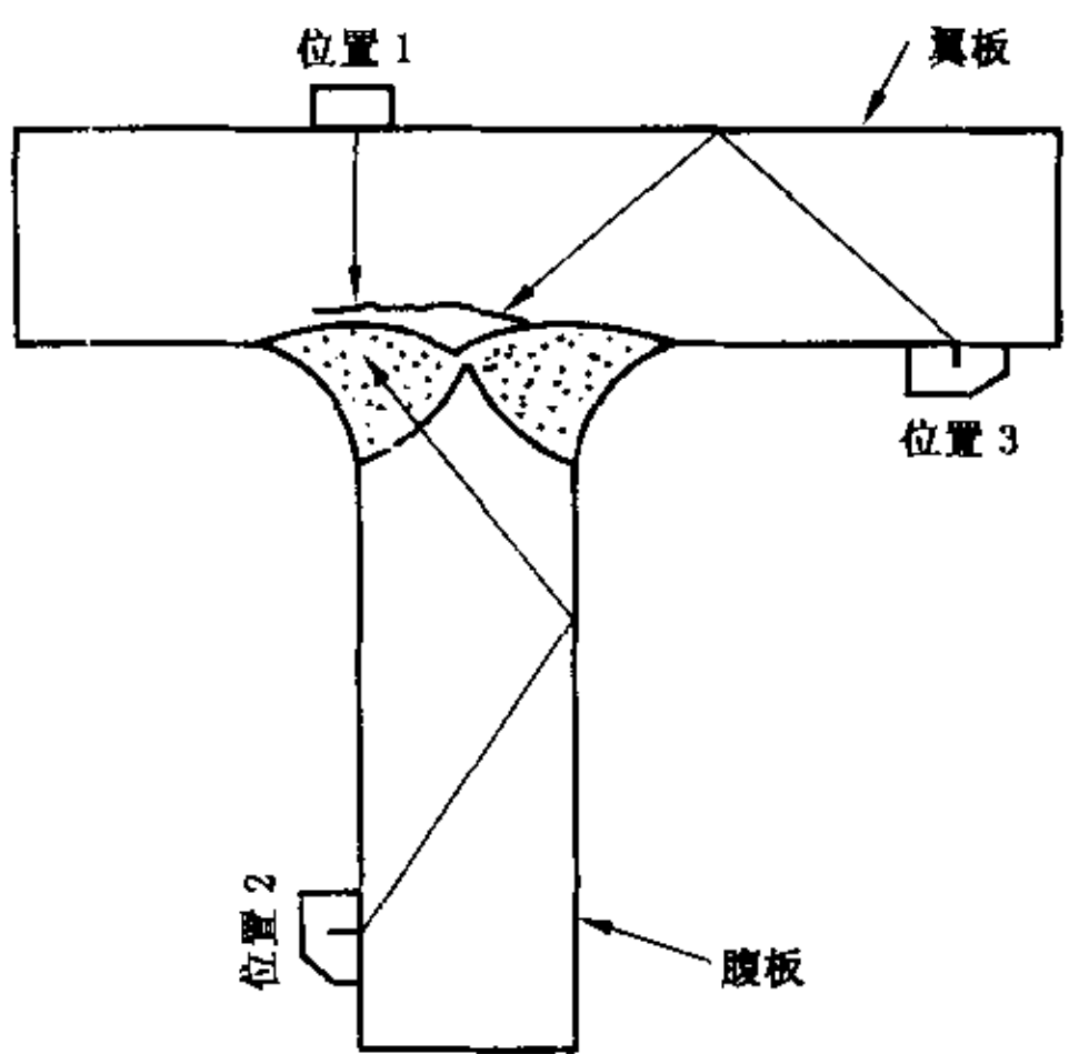
图 15 T 型接头
