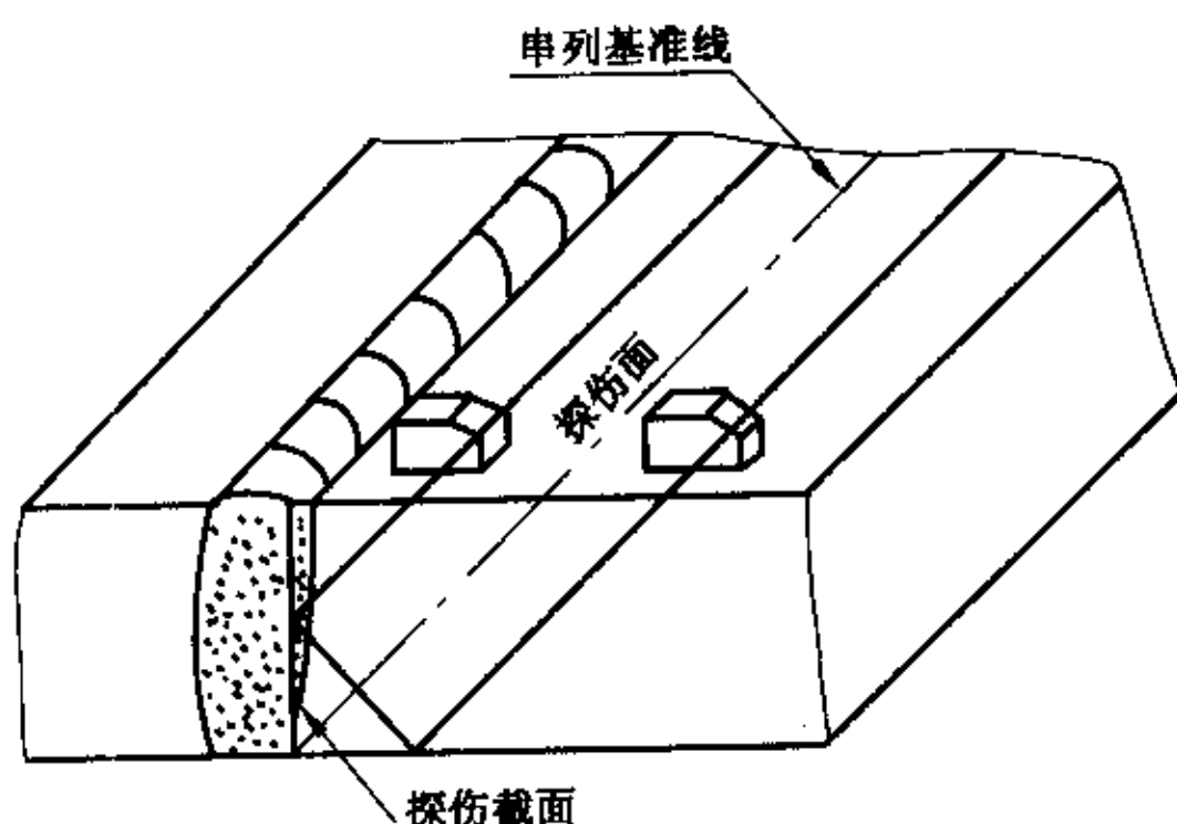
图 2 探伤截面及串列基准线
