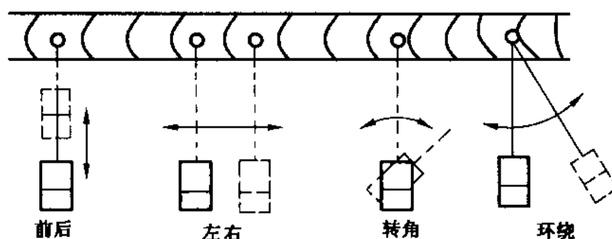
图 14 四种基本扫查方法
