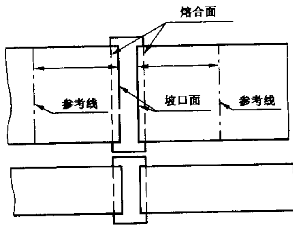
图 3 参考线
