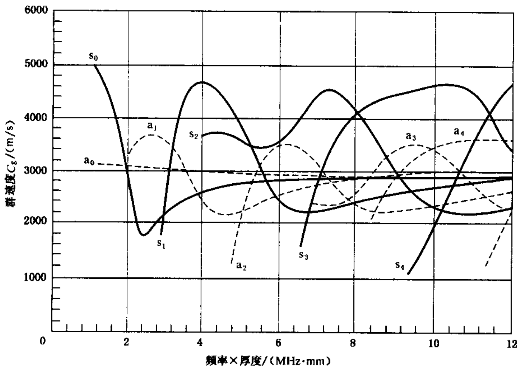
图 E2 1Cr18Ni9Ti 材料 Lamb 波群速度曲线
