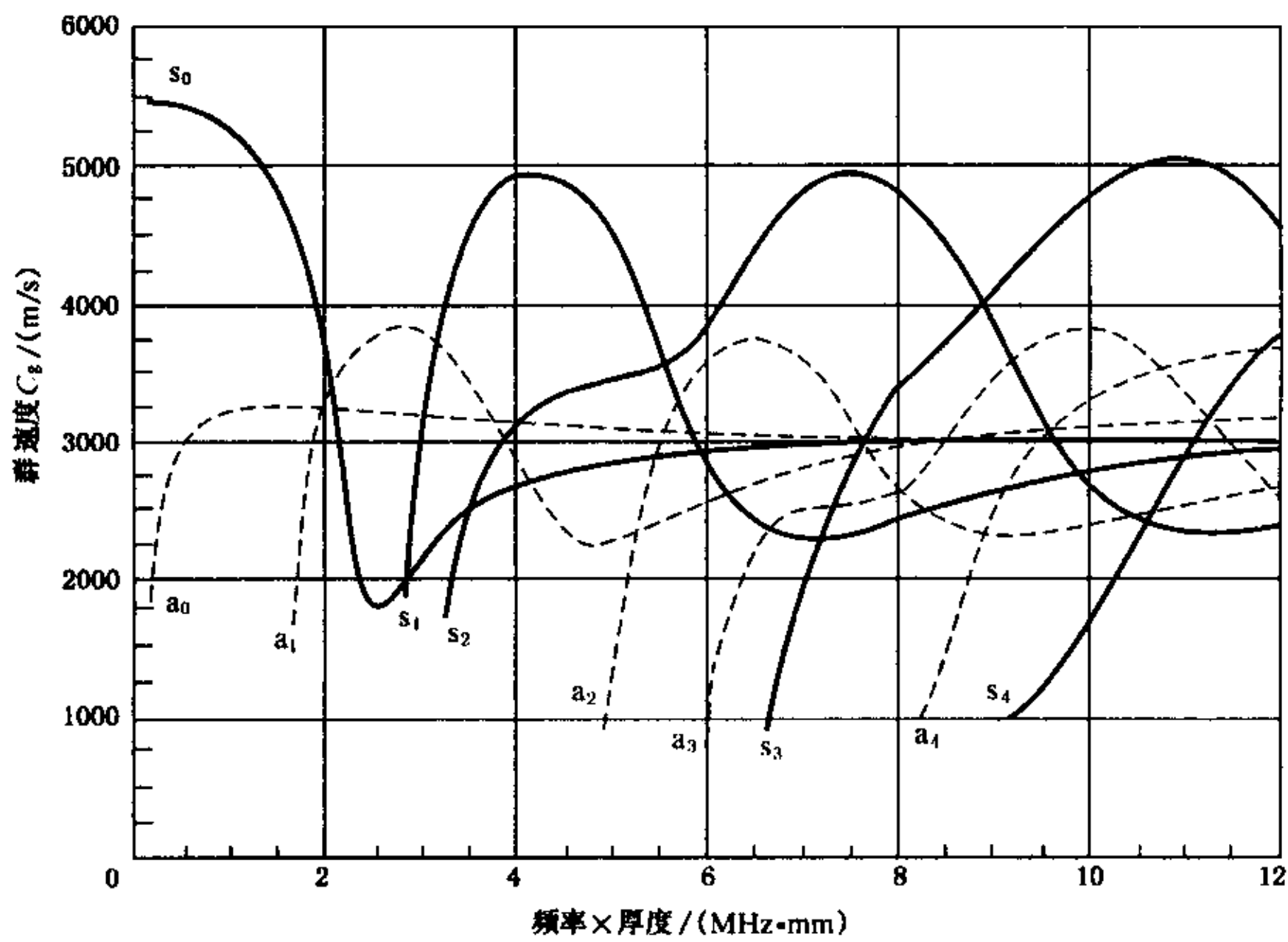
图 C2 低碳钢板 Lamb 波群速度曲线
