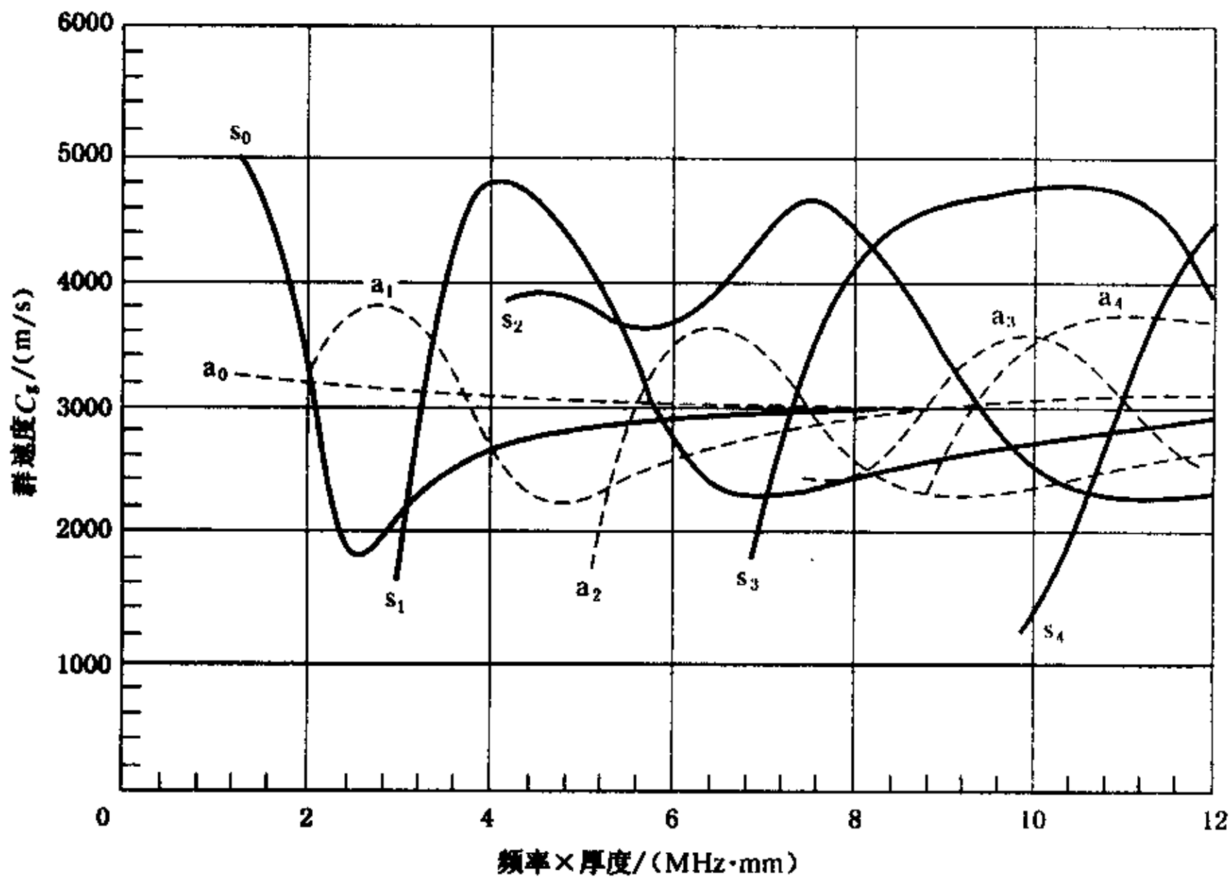
图 D2 1Cr13 材料 Lamb 波群速度曲线
