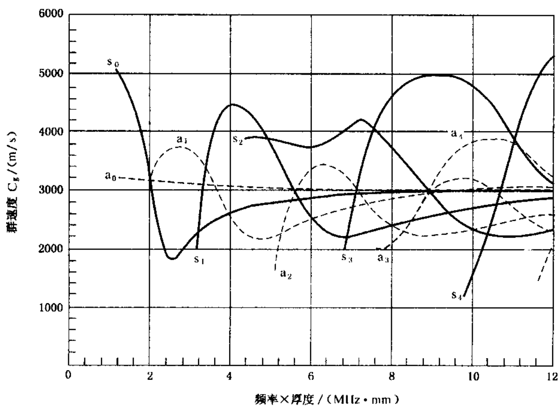
图 K2 TC4 材料 Lamb 波群速度曲线
