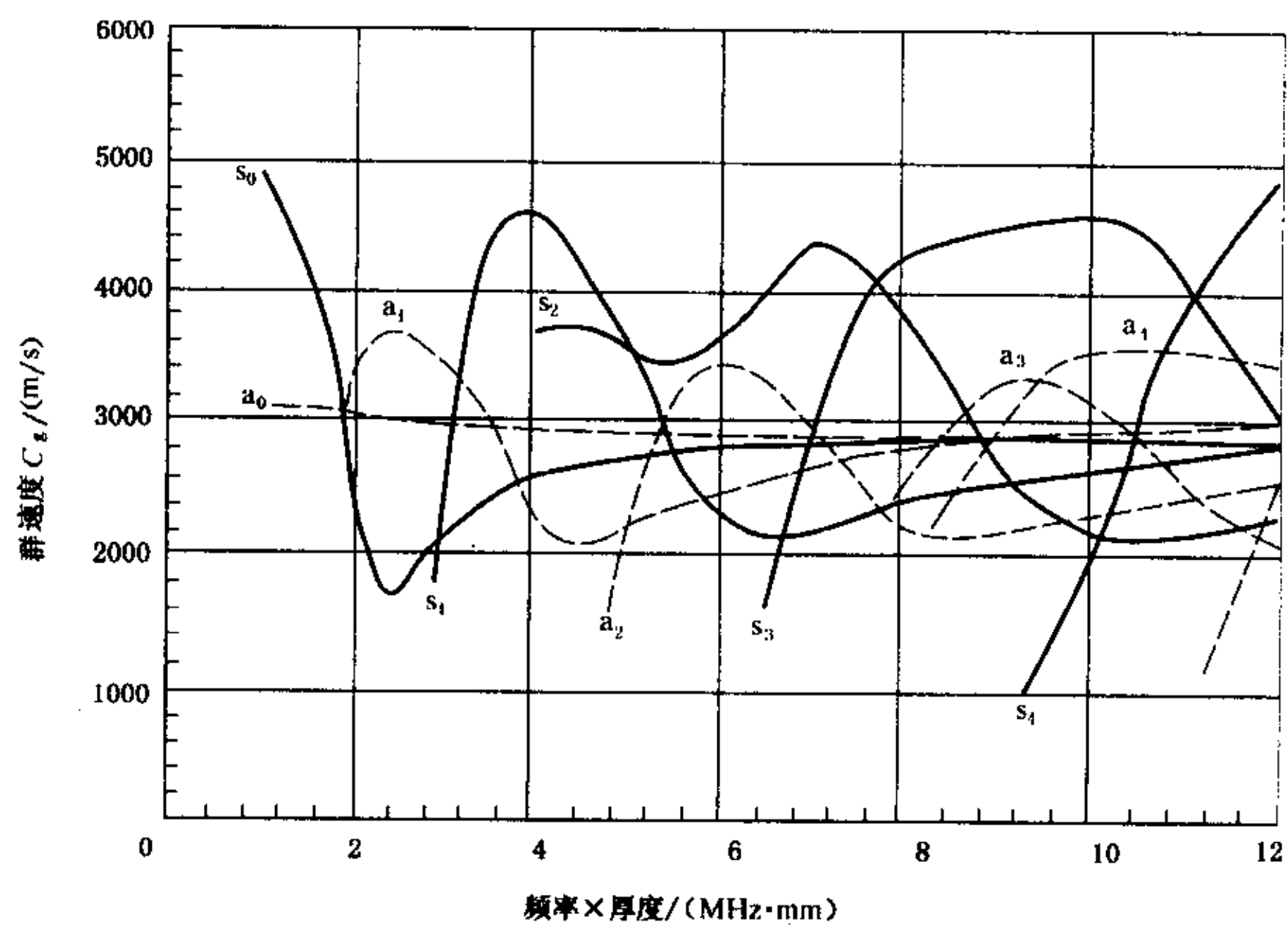
图 G2 GH169 材料 Lamb 波群速度曲线
