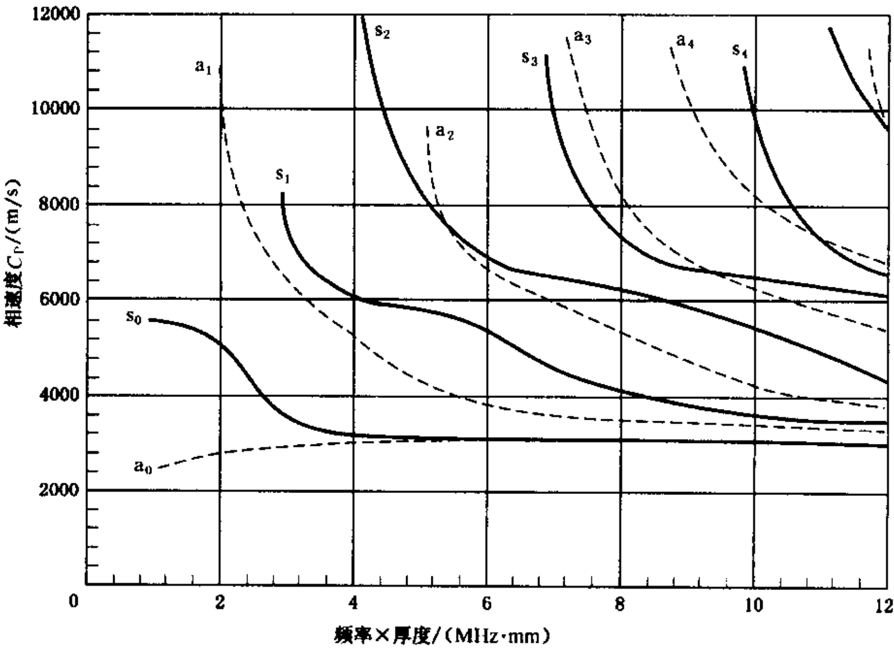
图 F1 Cr17Ni2 材料 Lamb 波相速度曲线
