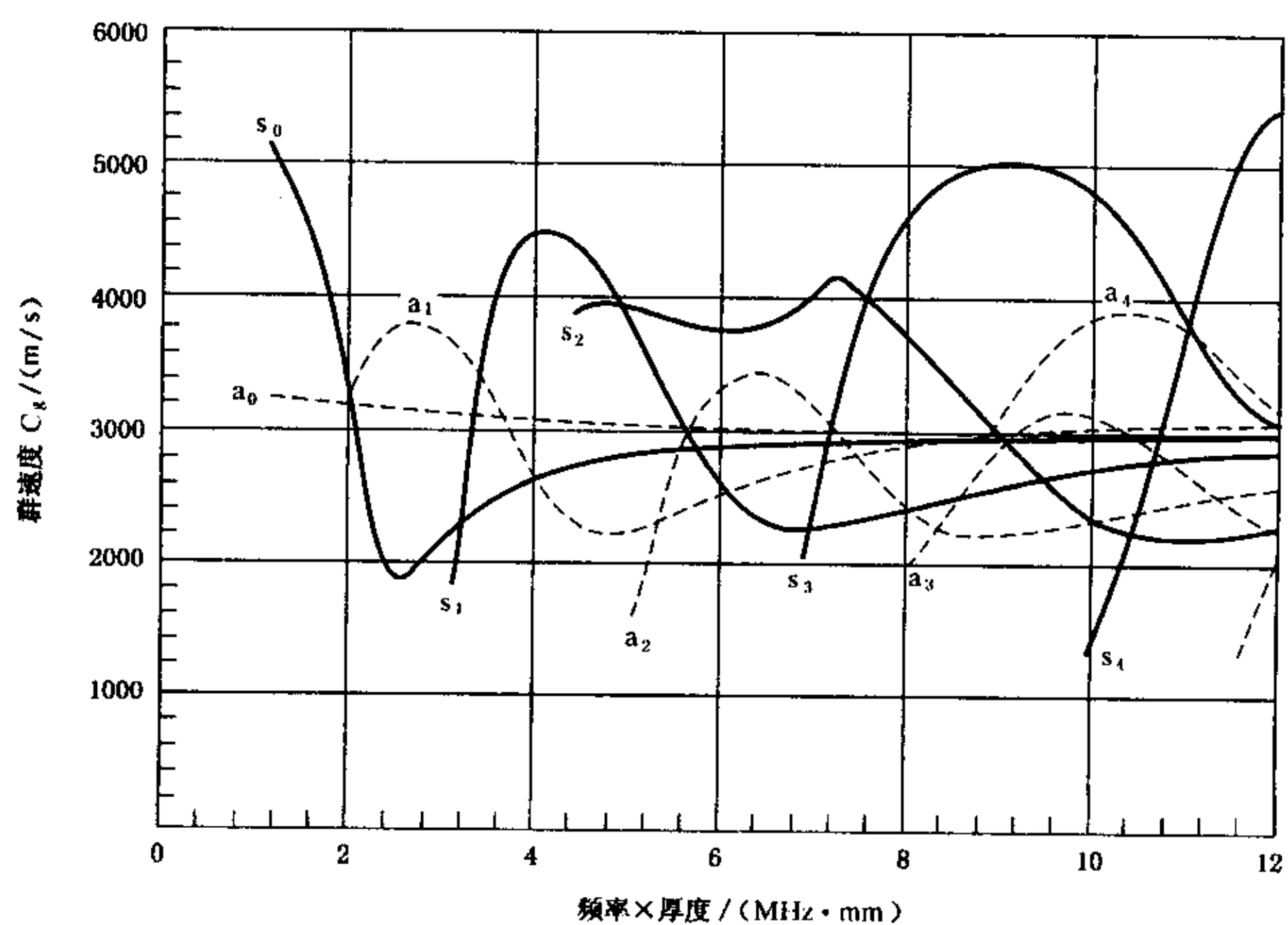
图 L2 5A06 材料 Lamb 波群速度曲线
