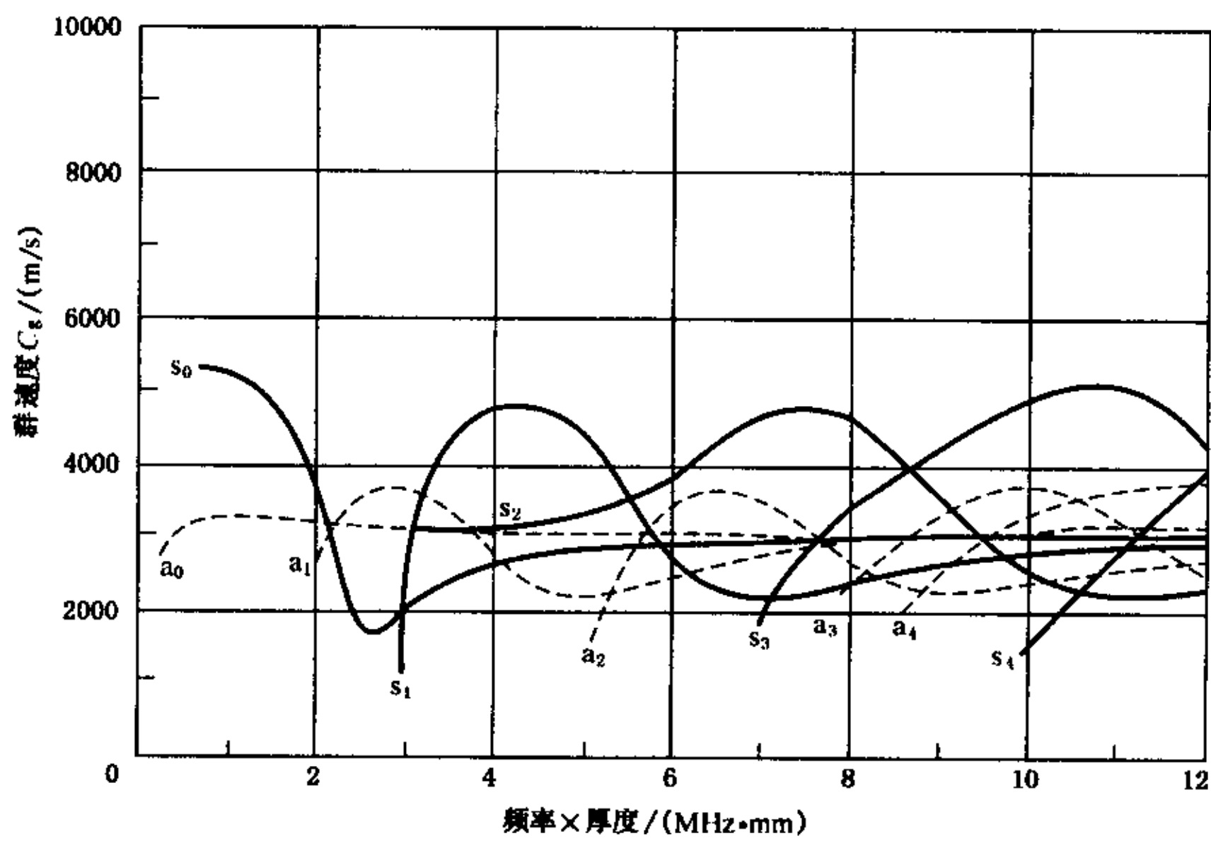
图 B2 406 钢板 Lamb 波群速度曲线
