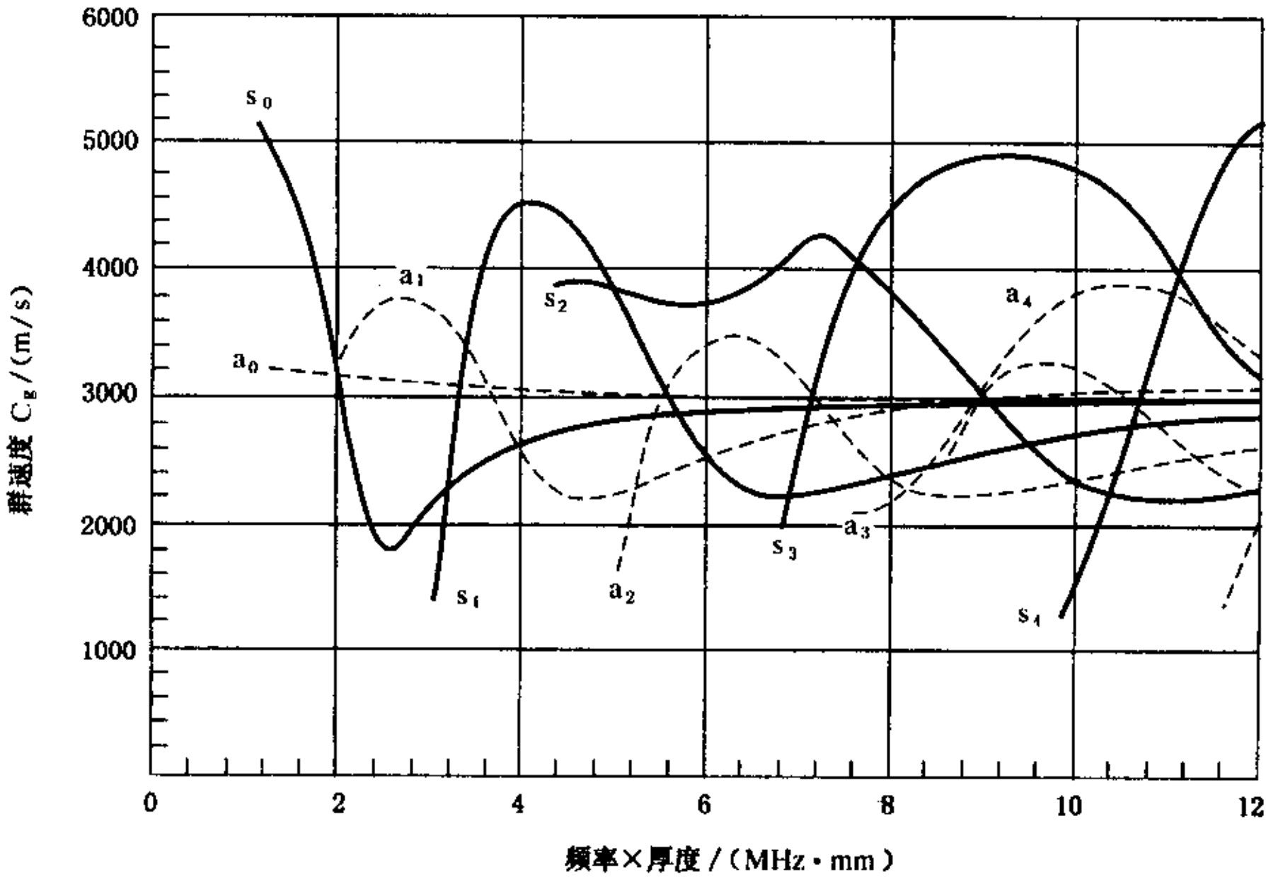
图 M2 2A12 材料 Lamb 波群速度曲线
