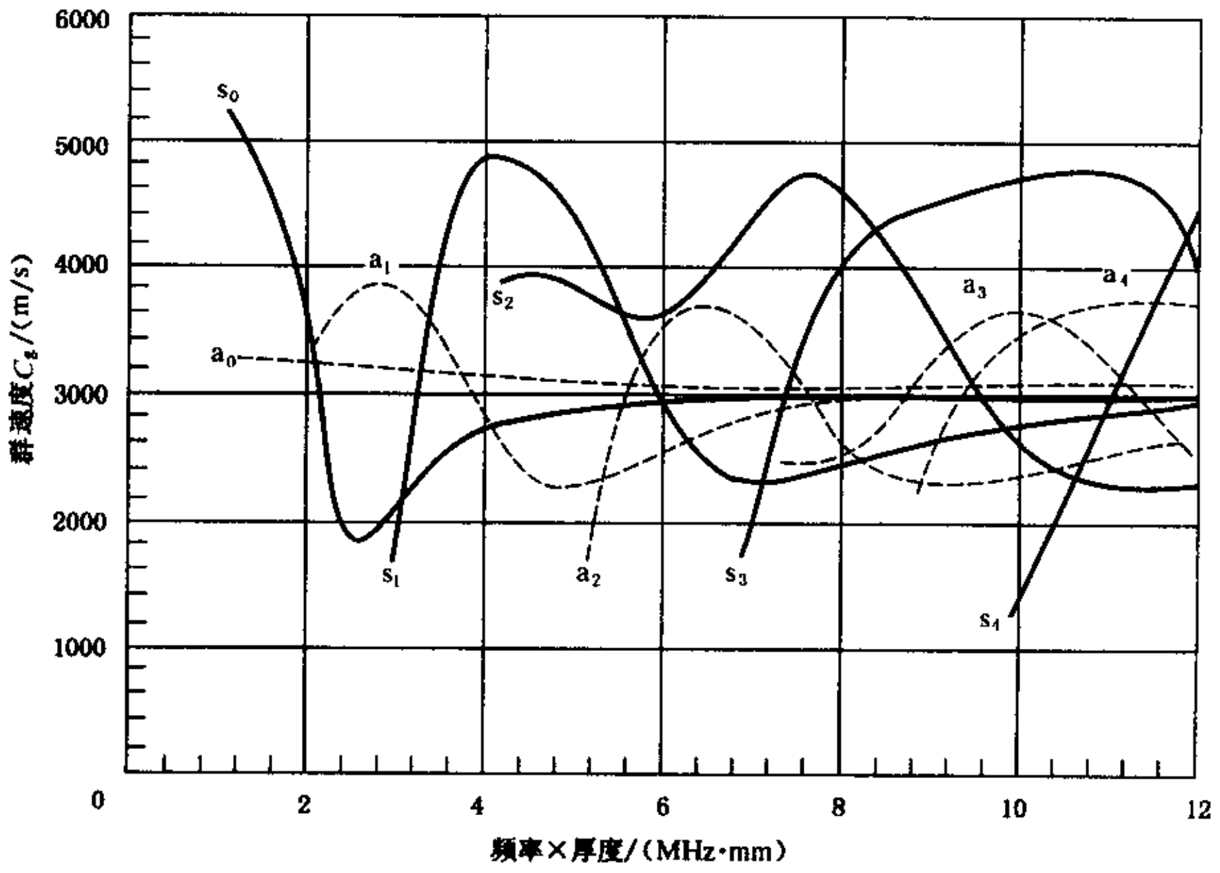
图 F2 Cr17Ni2 材料 Lamb 波群速度曲线
