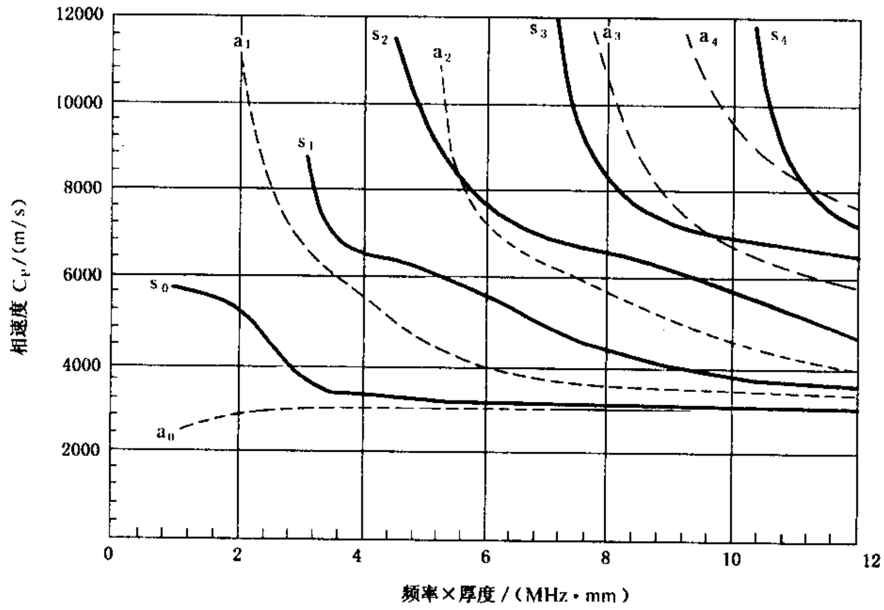
图 I1 TA7 材料 Lamb 波相速度曲线
