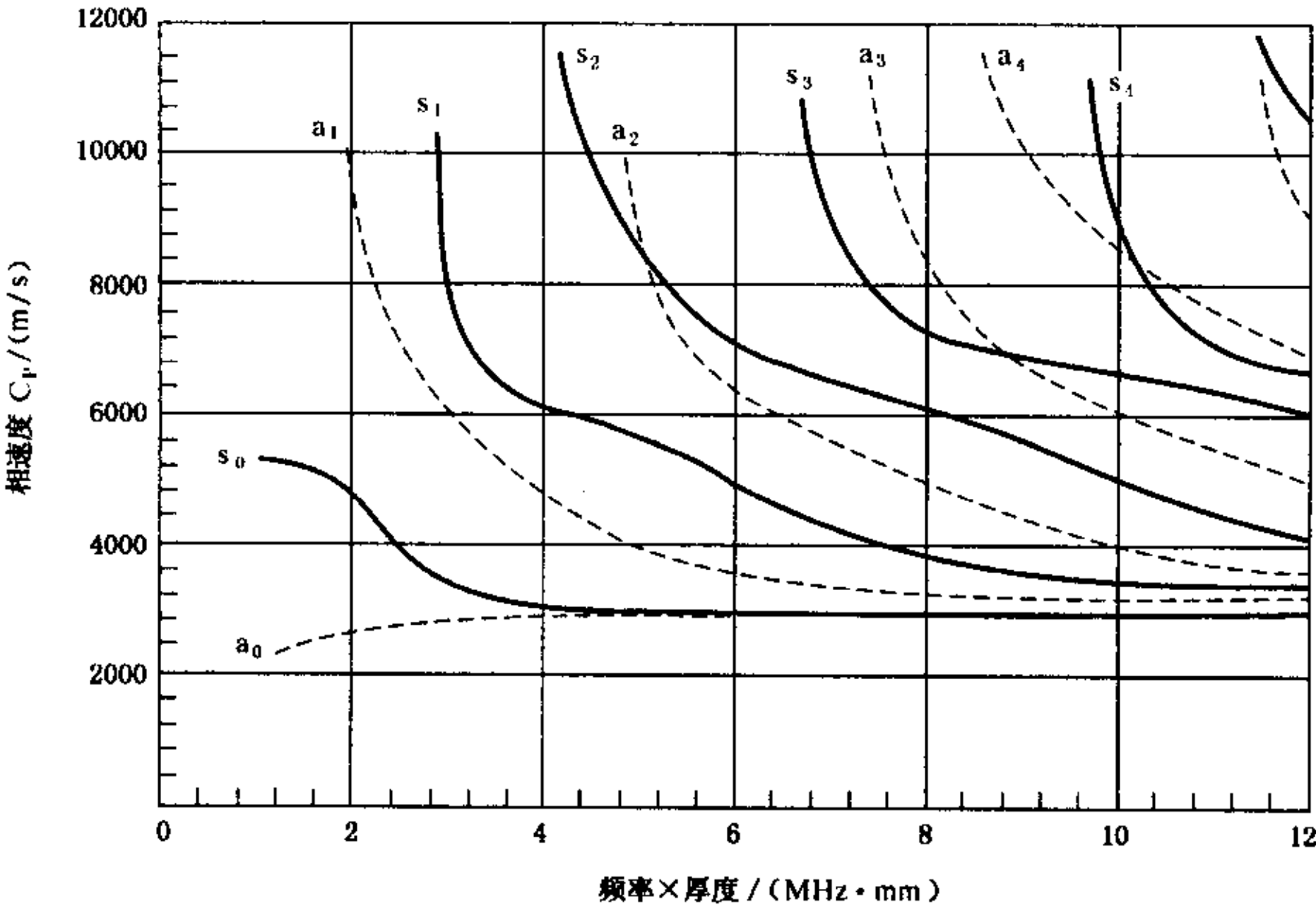
图 M1 2A12 材料 Lamb 波相速度曲线
