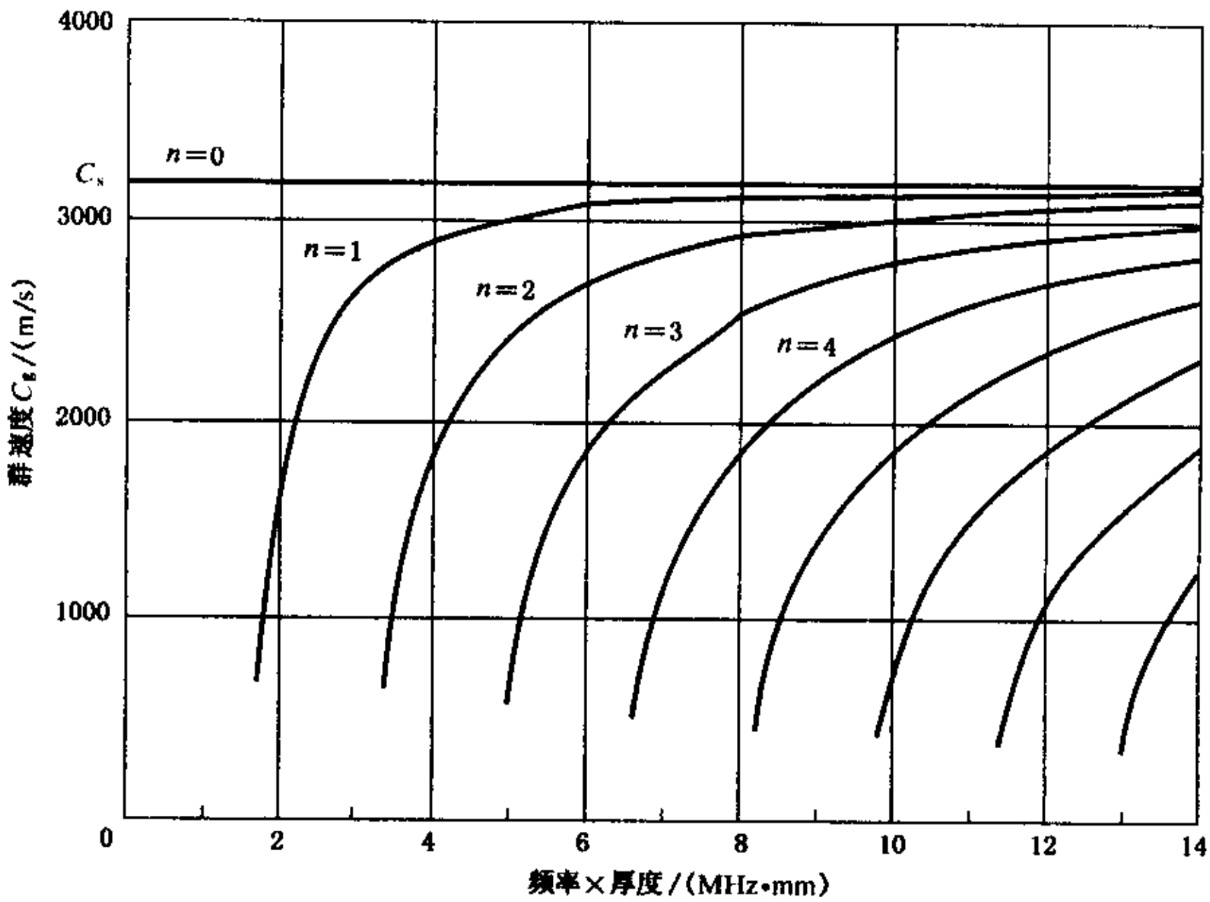
图 B4 406 钢板 SH 波群速度曲线
