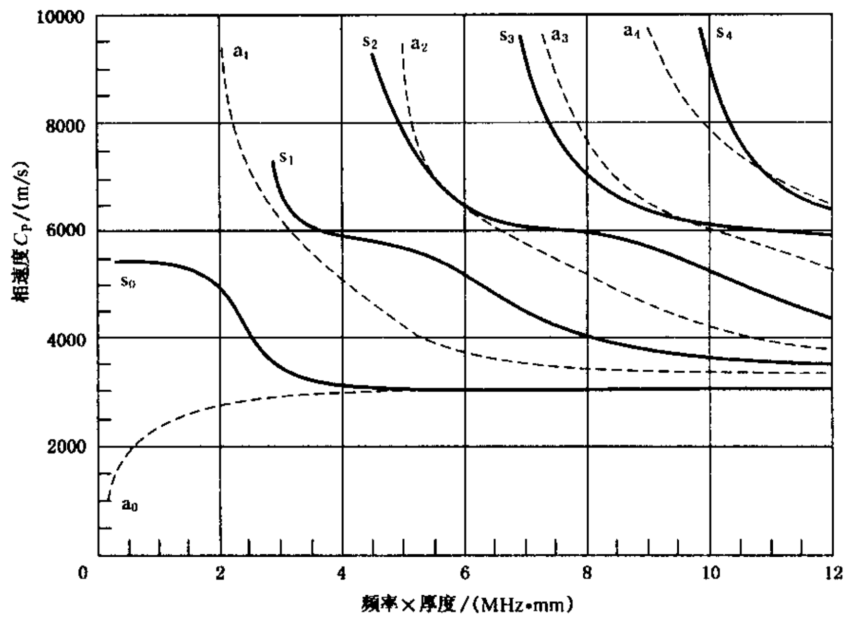
图 C1 低碳钢板 Lamb 波相速度曲线
