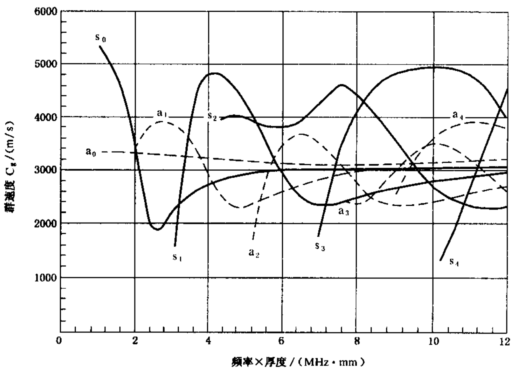
图 J2 TC2 材料 Lamb 波群速度曲线
