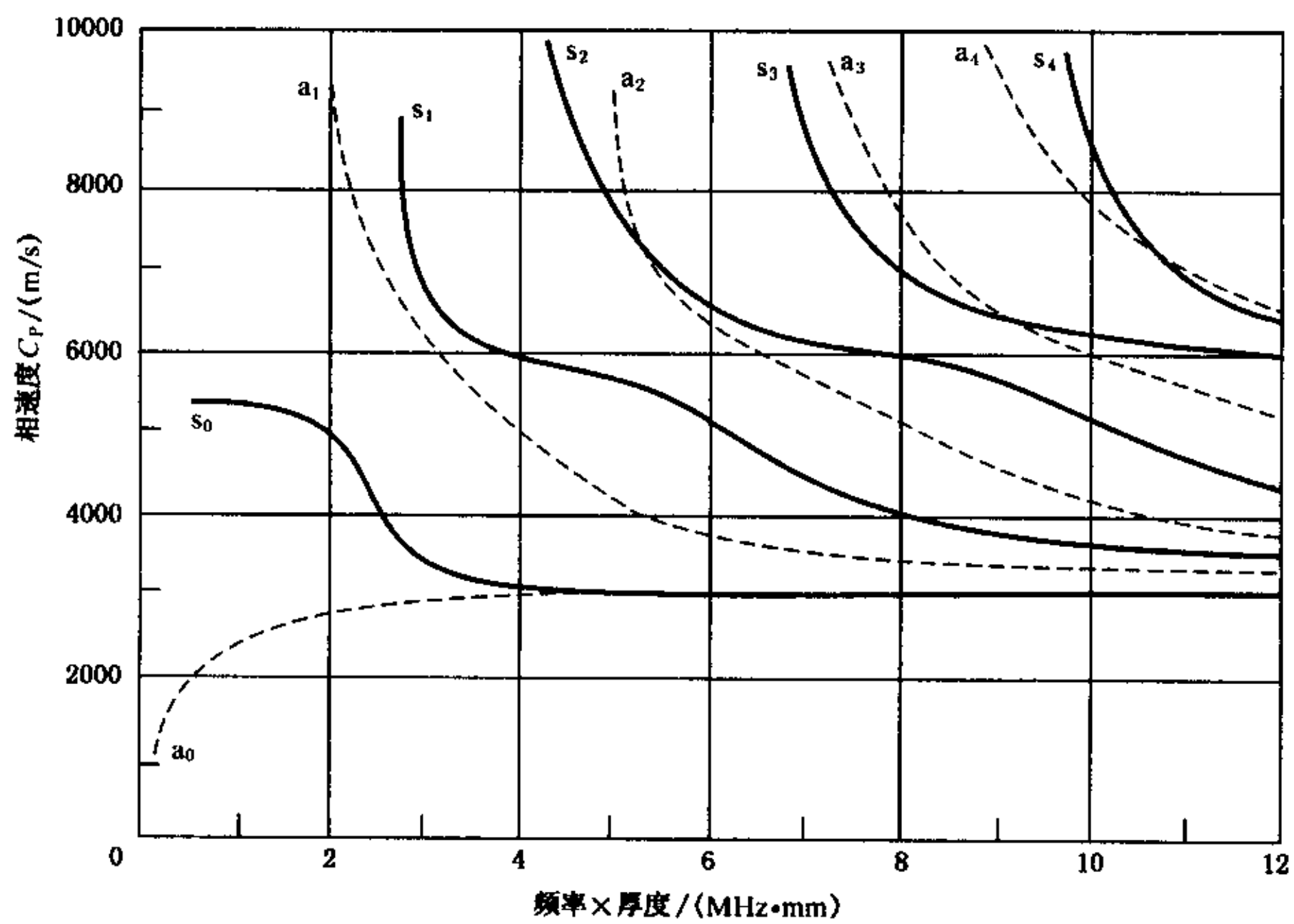
图 B1 406 钢板 Lamb 波相速度曲线
