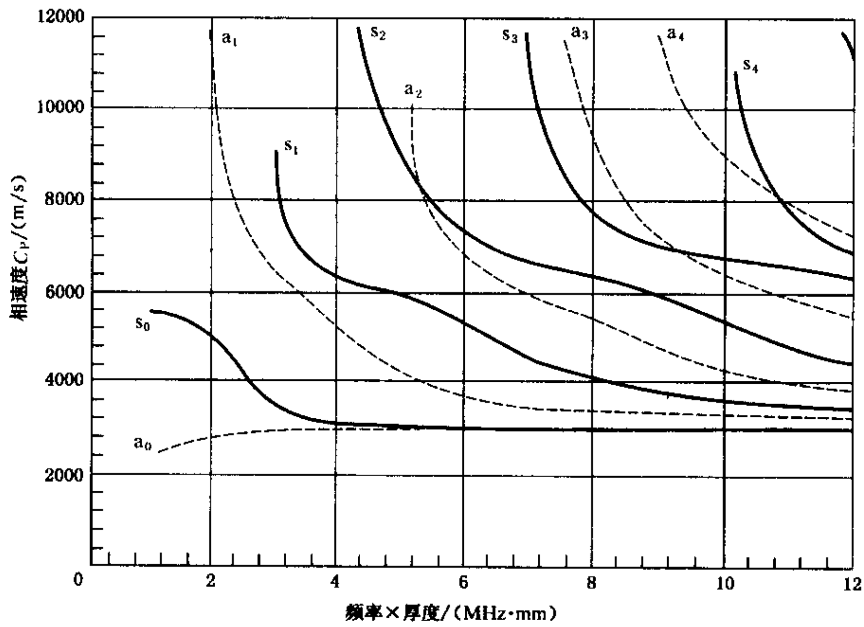
图 E1 1Cr18Ni9Ti 材料 Lamb 波相速度曲线
