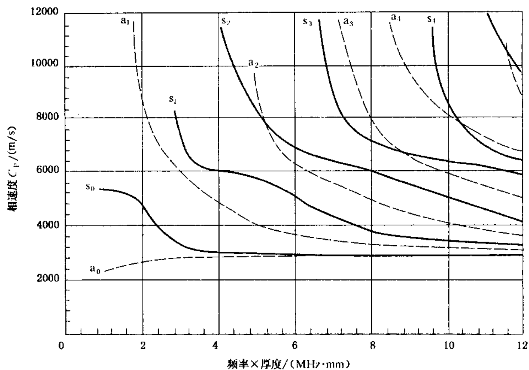
图 H1 TA2 材料 Lamb 波相速度曲线
