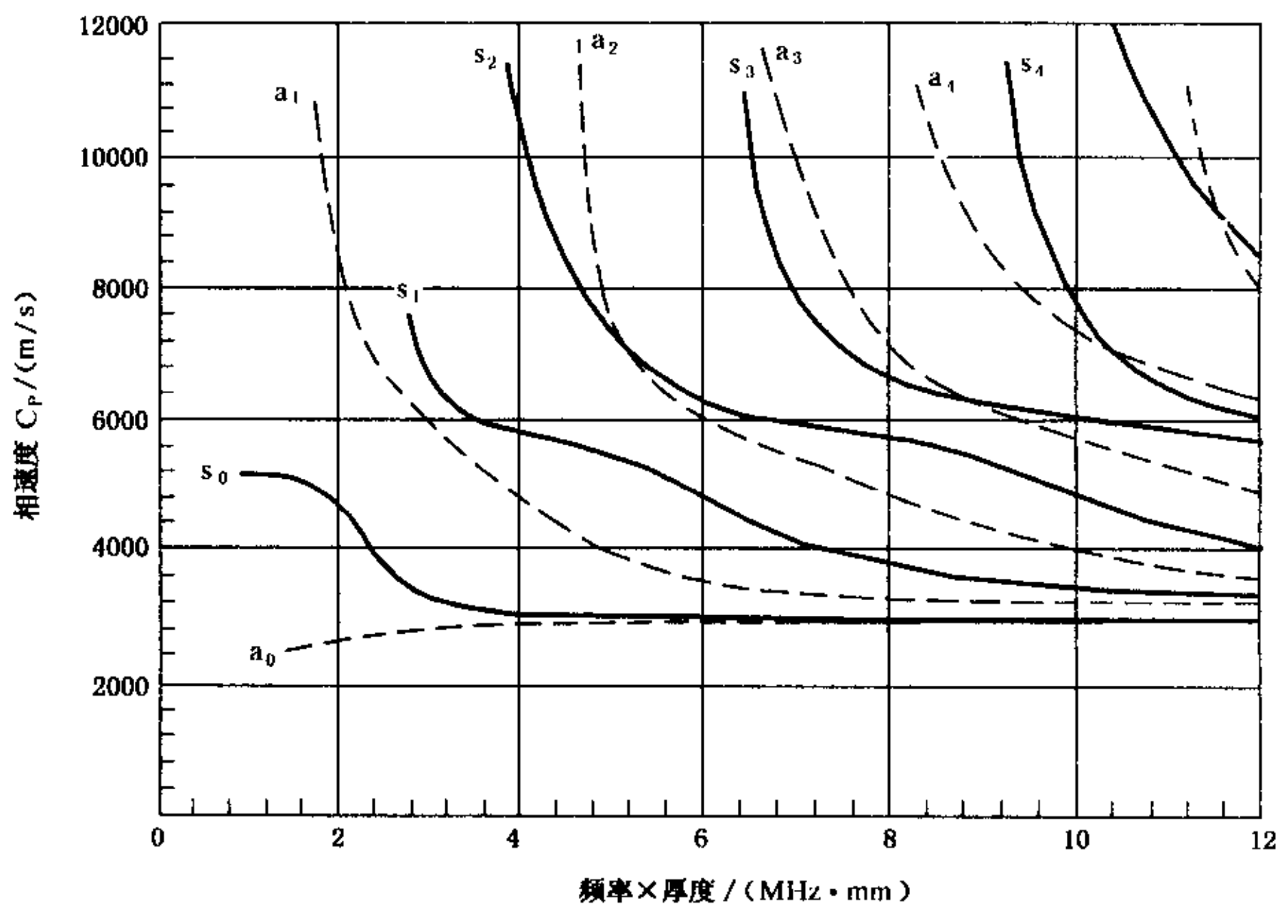
图 J1 TC2 材料 Lamb 波相速度曲线
