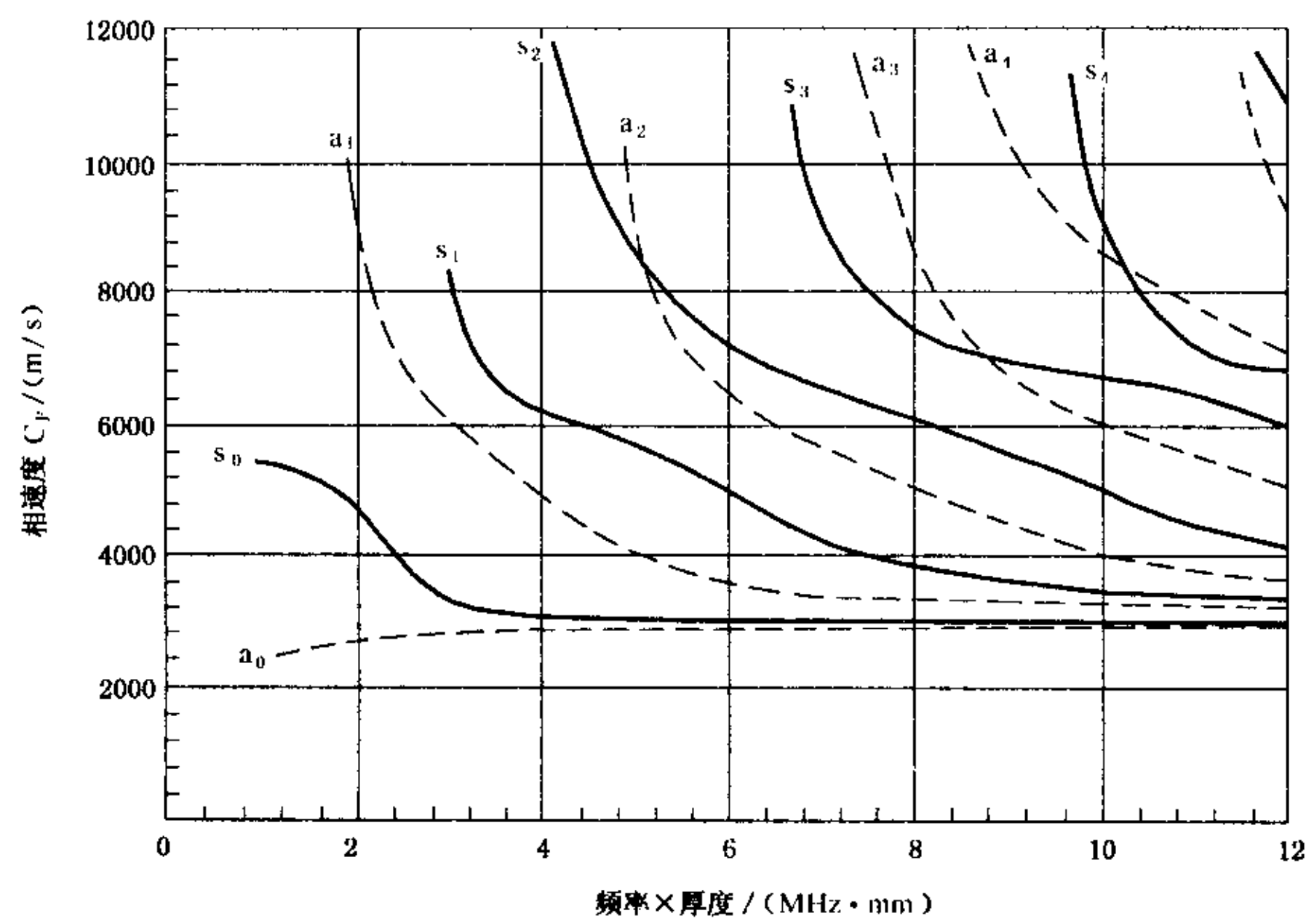
图 K1 TC4 材料 Lamb 波相速度曲线
