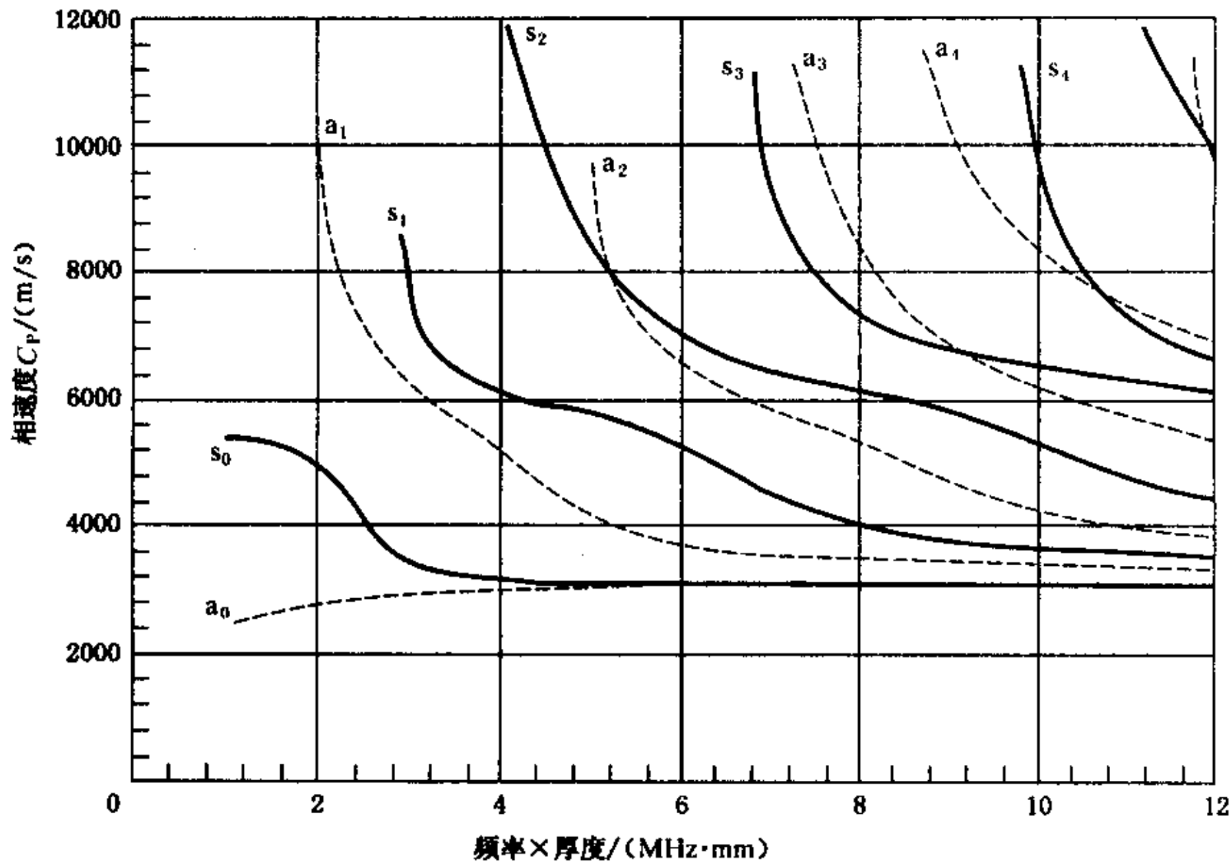
图 D1 1Cr13 材料 Lamb 波相速度曲线
