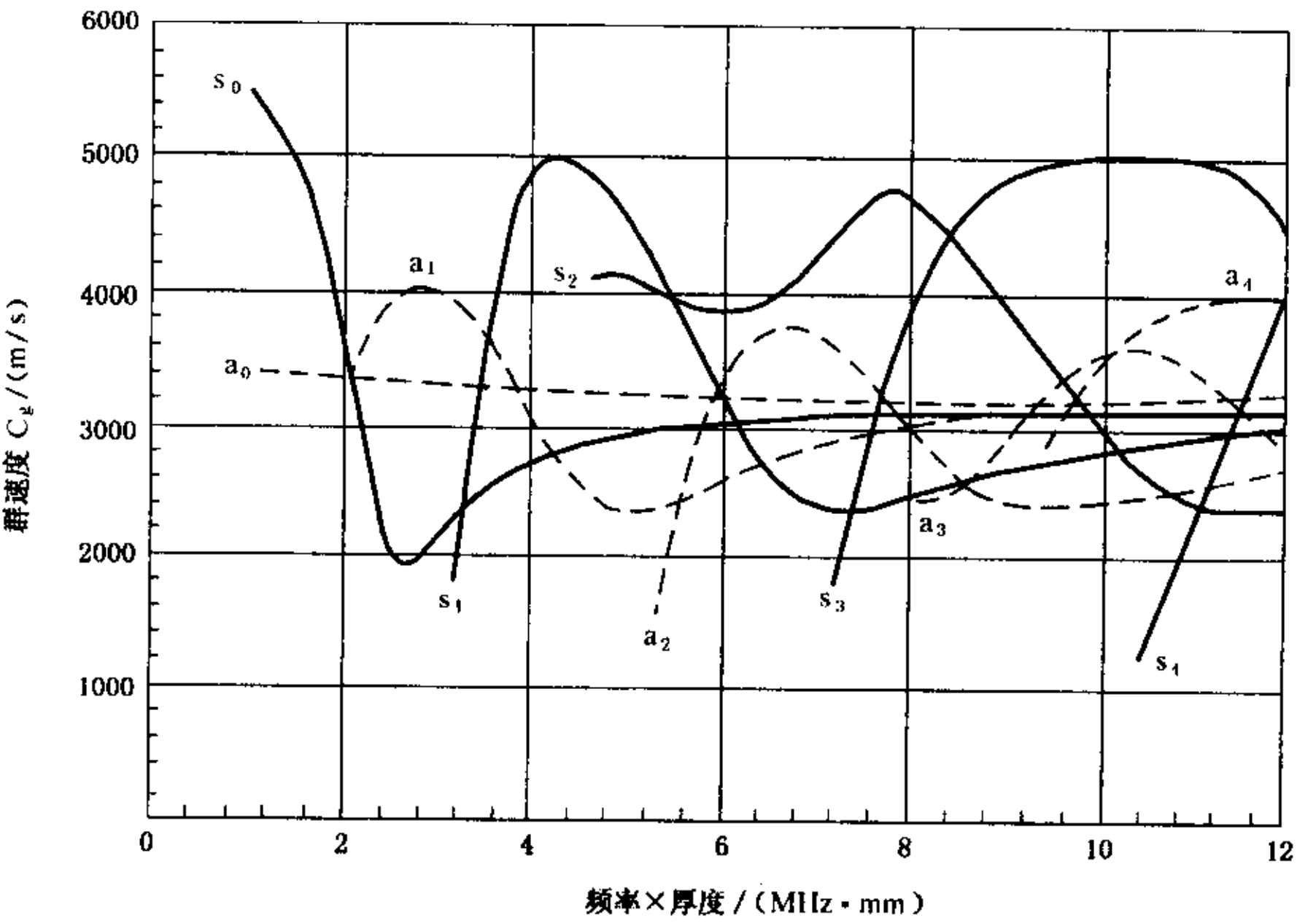
图 I2 TA7 材料 Lamb 波群速度曲线
