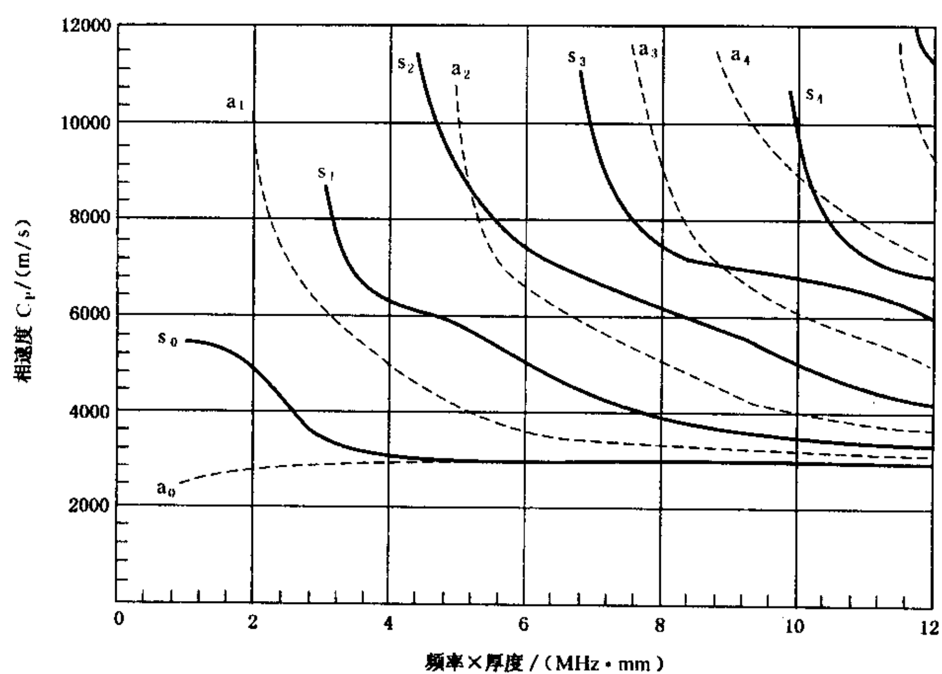
图 L1 5A06 材料 Lamb 波相速度曲线
