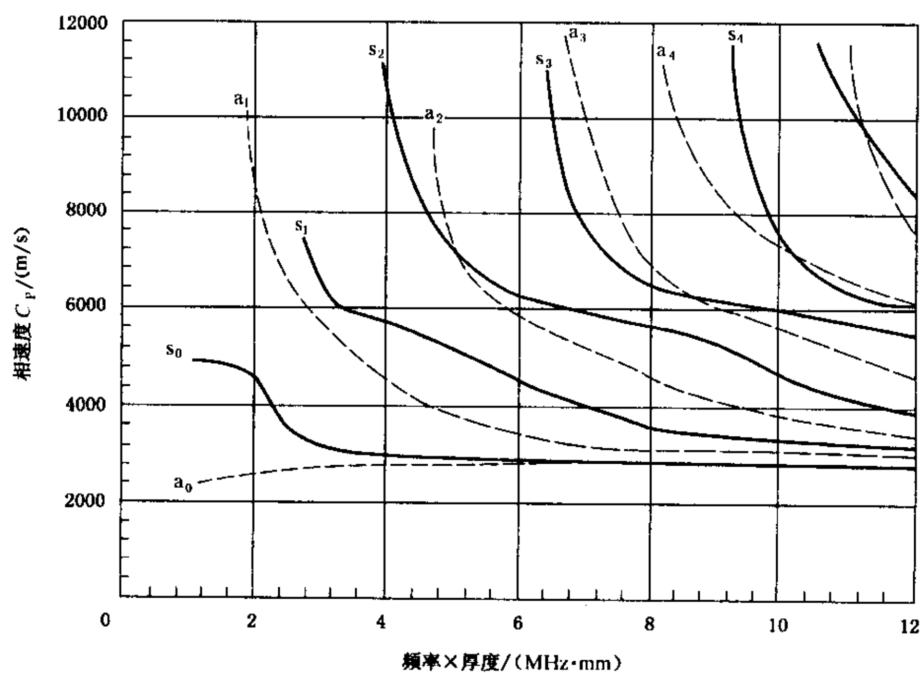
图 G1 GH169 材料 Lamb 波相速度曲线
