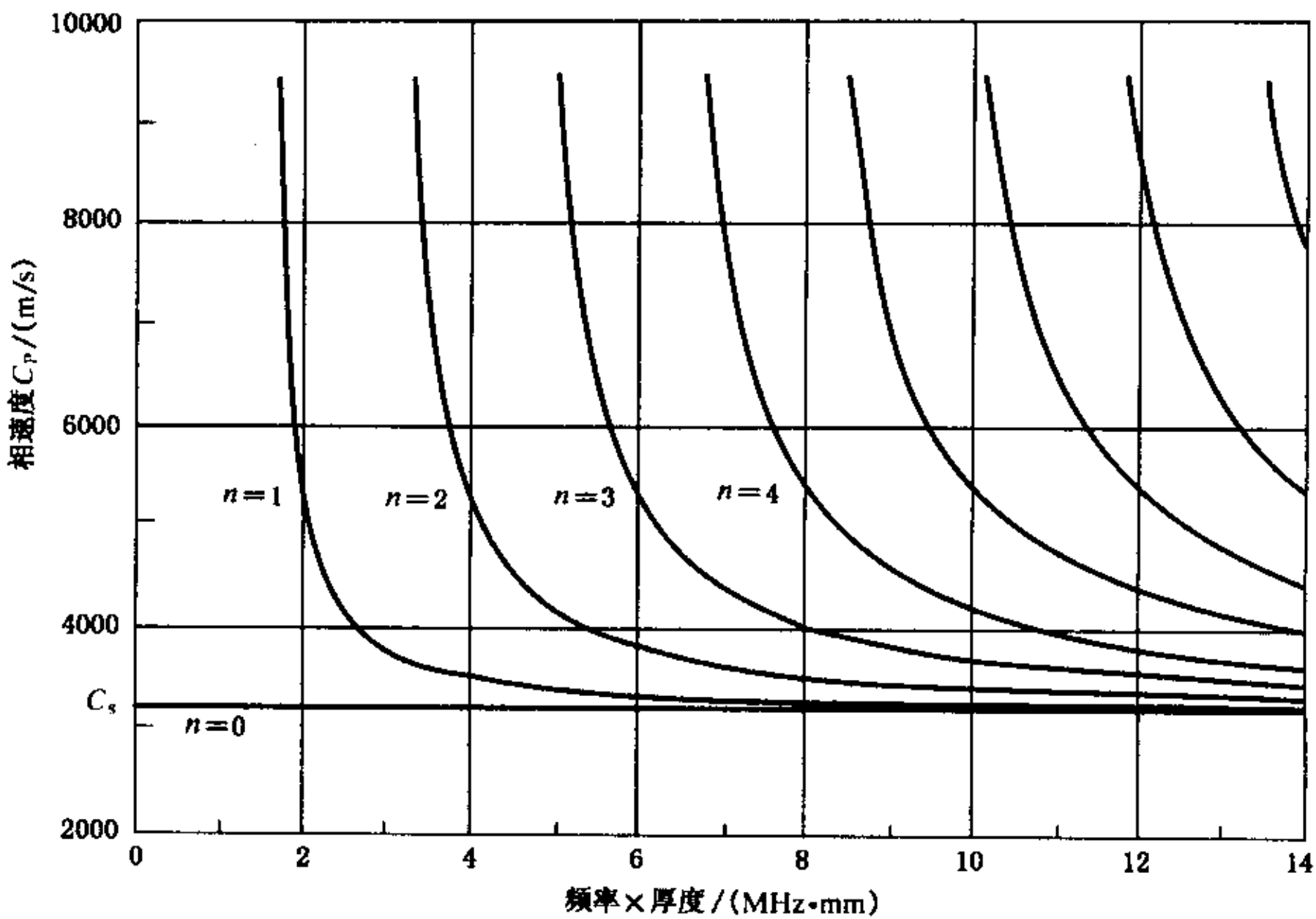
图 B3 406 钢 SH 波相速度曲线
