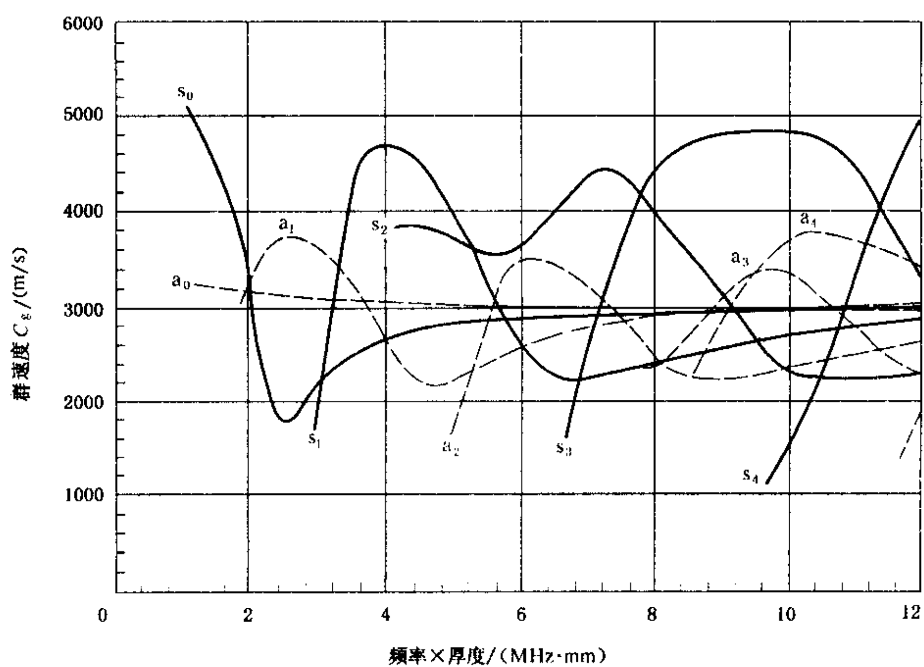
图 H2 TA2 材料 Lamb 波群速度曲线
