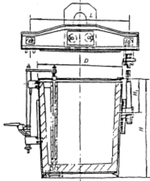
图2 不带手动倾翻机构小型盛钢桶
