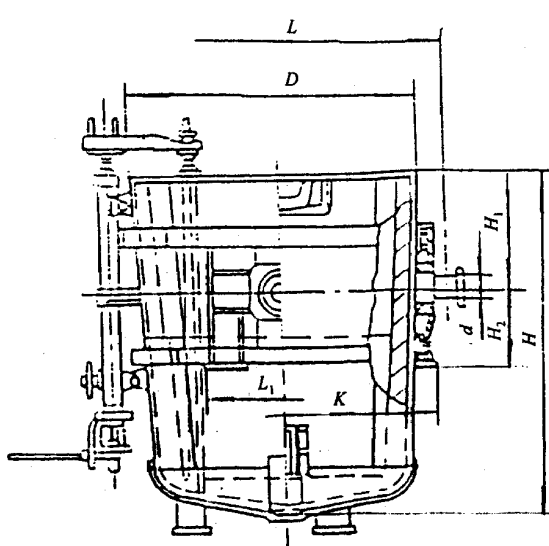
图3 中型盛钢桶
