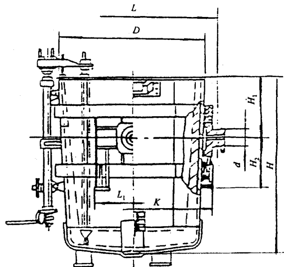
图4 大型盛钢桶
